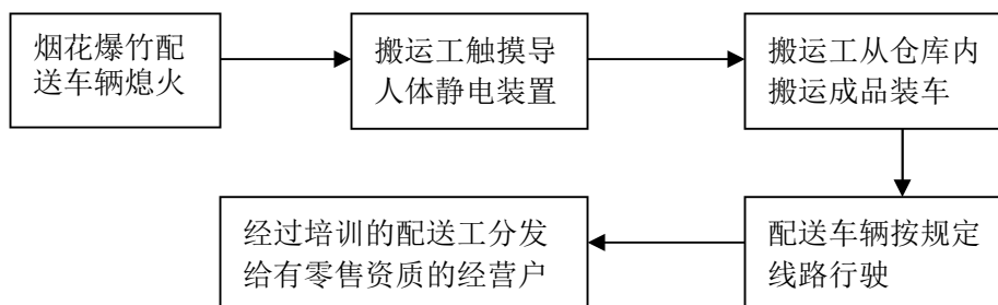
图 2.4-2 烟花爆竹配送工艺流程示意框图
