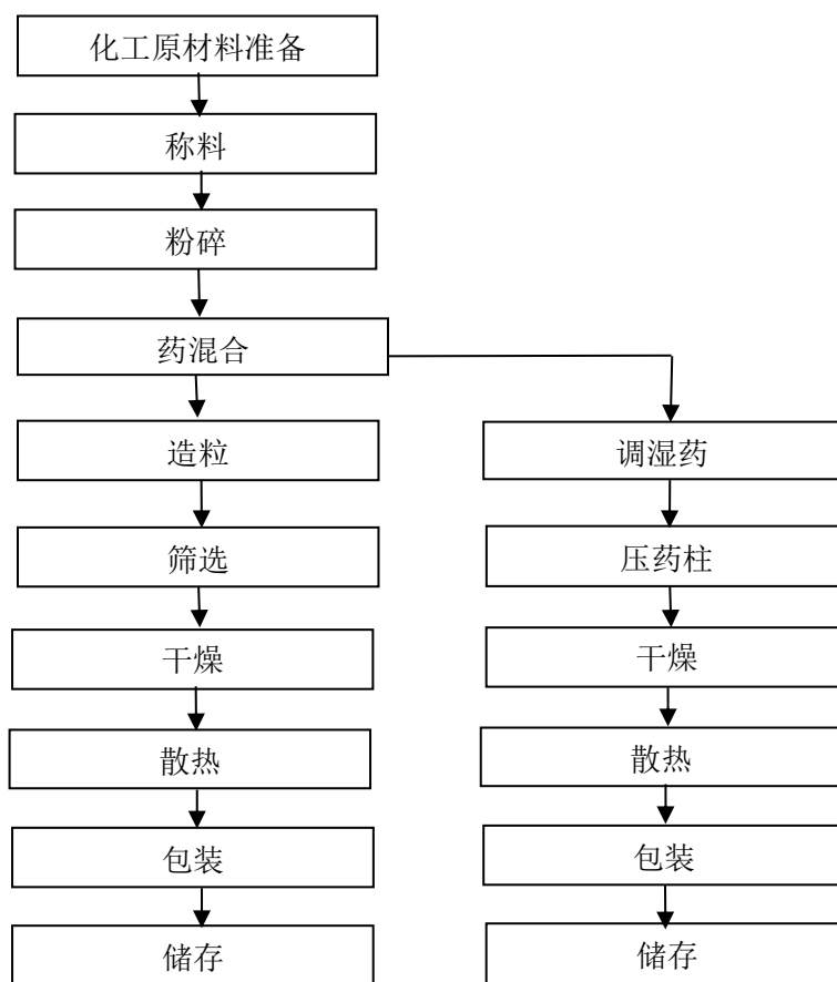
图 2.4-1 亮珠、药柱生产工艺流程图
