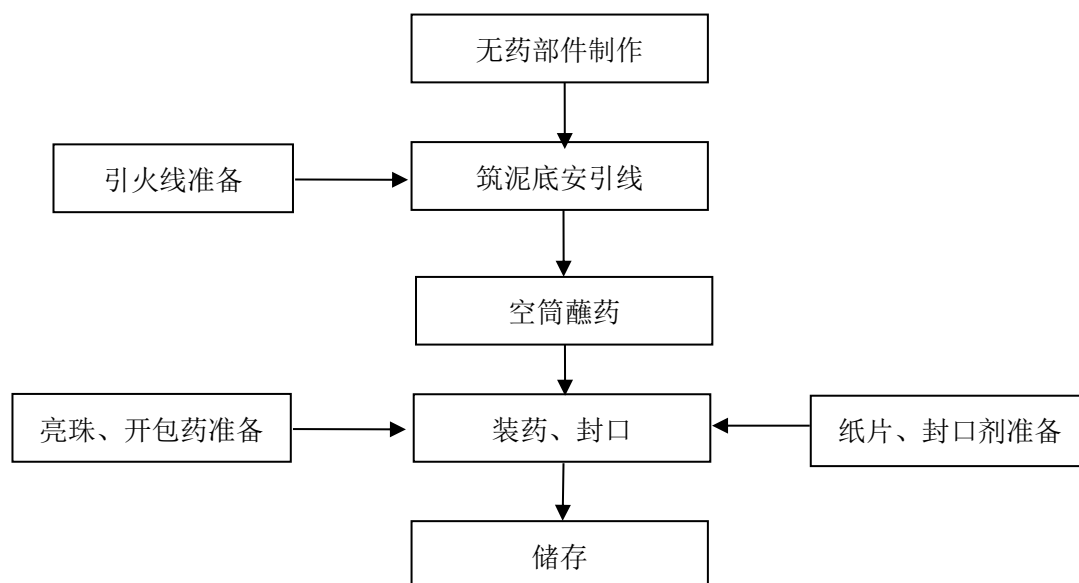
图 2.4-2 效果内筒（一）生产工艺流程图
