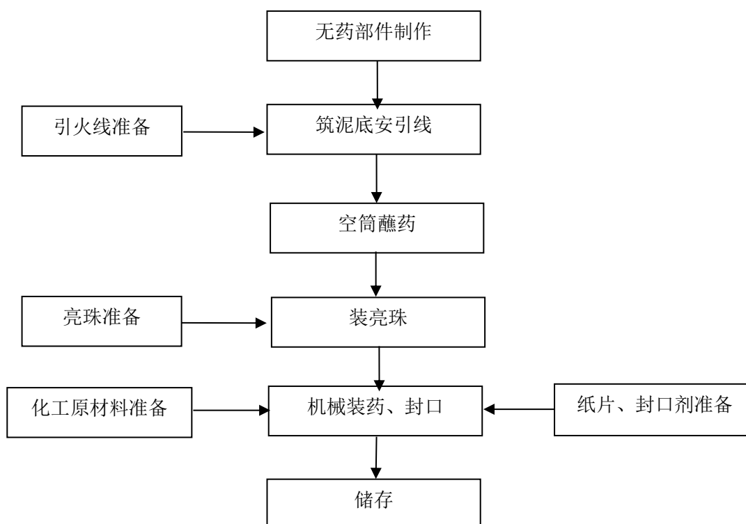
图 2.4-3 效果内筒（二）生产工艺流程图
