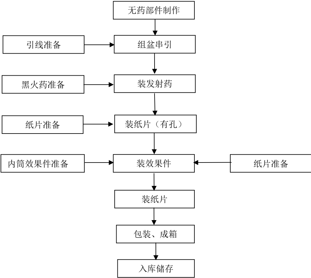
图 2.4-4 组合烟花类产品生产工艺流程图
